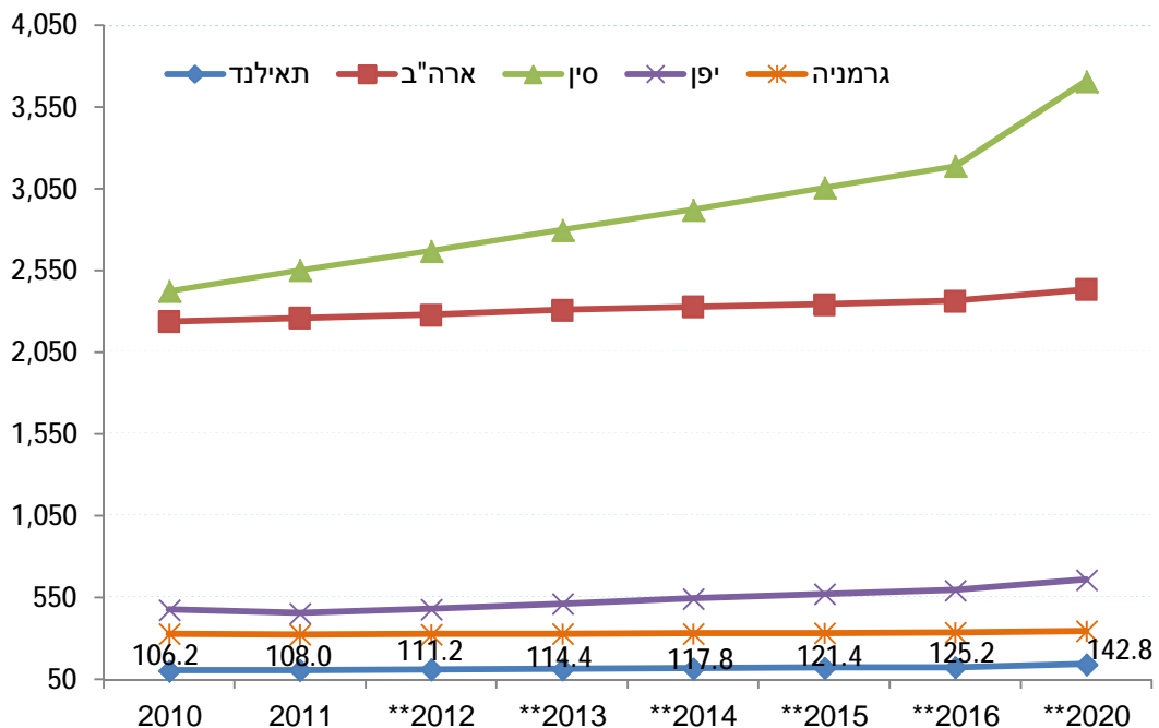
צריכת אנרגיה (שווה ערך למיליון טון נפט) בהשוואה עולמית (המספרים בתוך הגרף מתייחסים לתאילנד בלבד)
